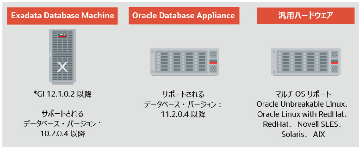
図2 : Oracle ACFSのプラットフォーム・サポート - オンプレミスのExadata、Oracle Database Appliance、および汎用ハードウェア
