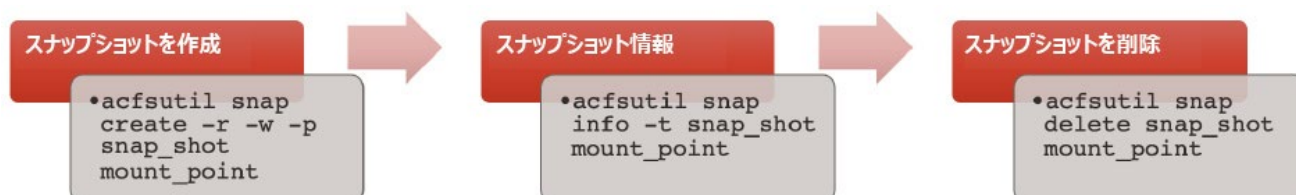
図7: Oracle ACFSスナップショット
