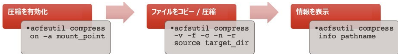
図6 : Oracle ACFS圧縮
