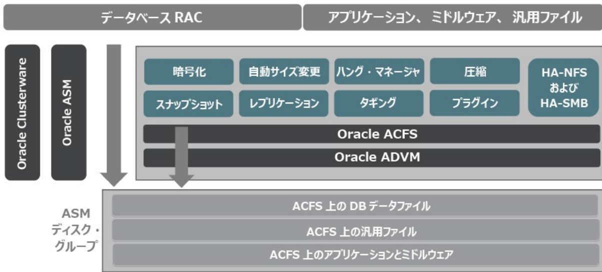
図1：Oracle ACFSのアーキテクチャ
