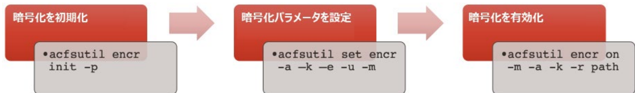
図5 : Oracle ACFS暗号化
