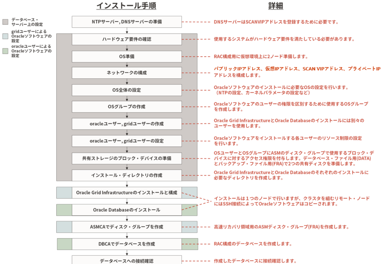
図 2 本ガイドで実行するインストール過程
