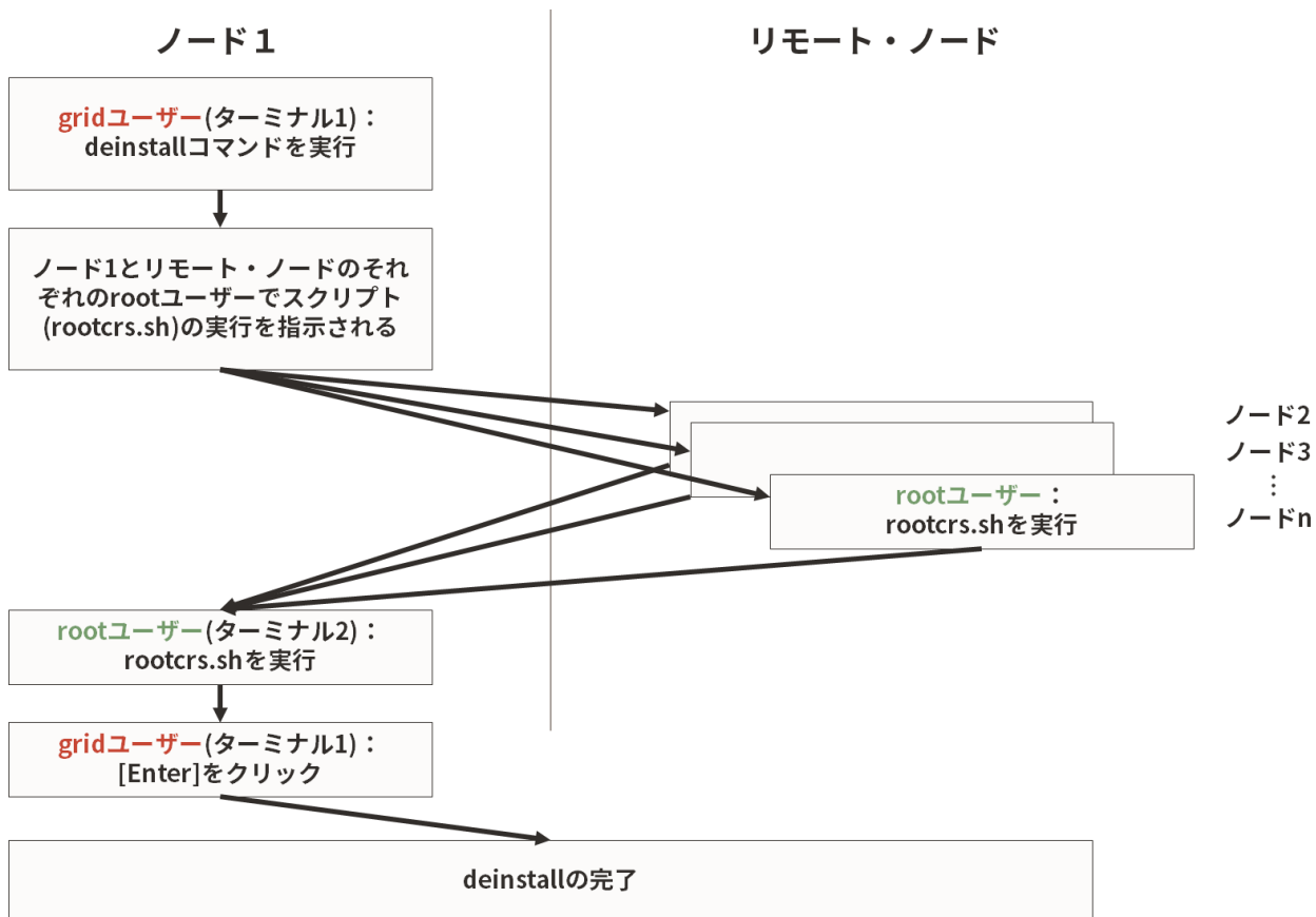
図 4 Oracle Grid Infrastructure の deinstall の過程
