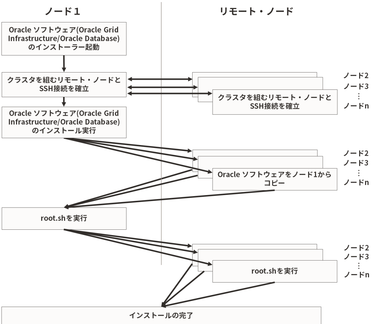
図 3 SSH 接続によるリモート・ノードへのインストール過程
