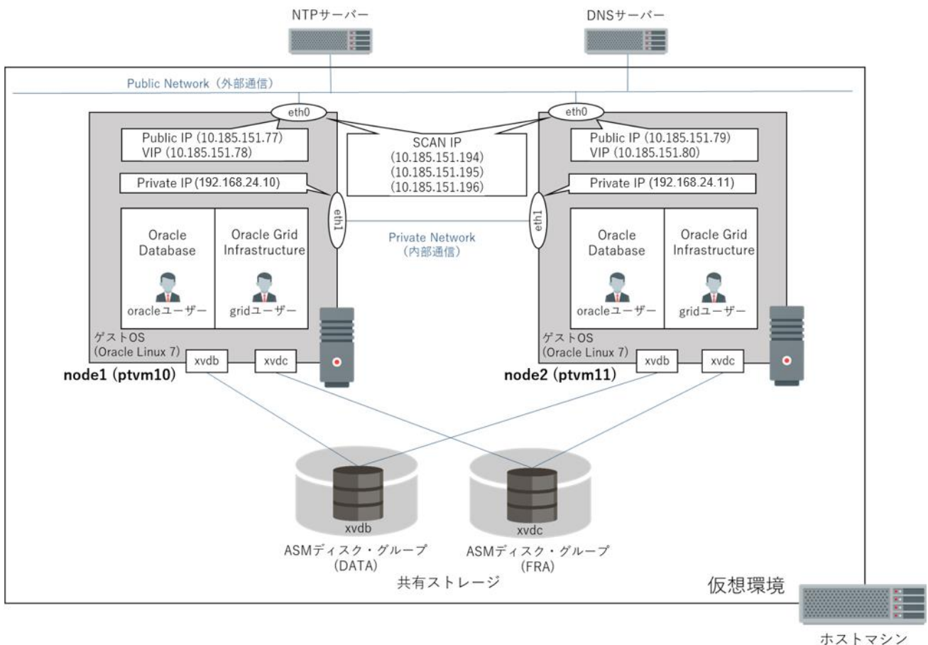
図 1 本ガイドのシステム構成図
