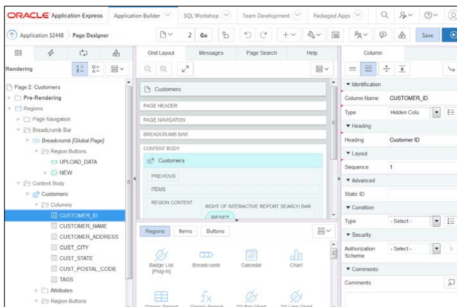
図2：Page Designerを使用したアプリケーション・ページの管理
